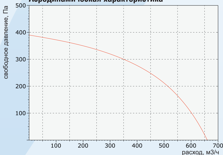
Аэродинамическая характеристика
